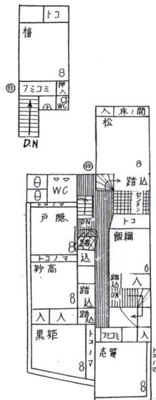
三階平面図
